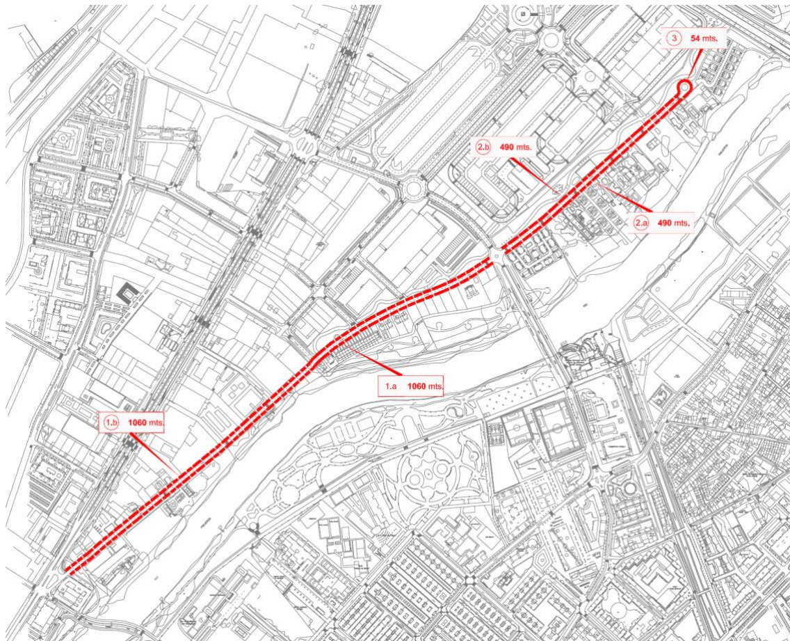
PLANO TRAMO A SEÑALIZAR CICLOCARRIL CAMINO DEL CABILDO
